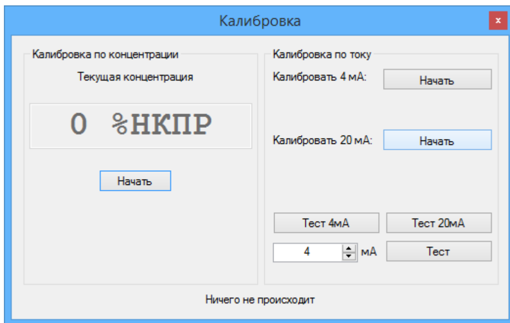
Рисунок Л.2- Окно калибровки газоанализатора по концентрации газа и по току.
