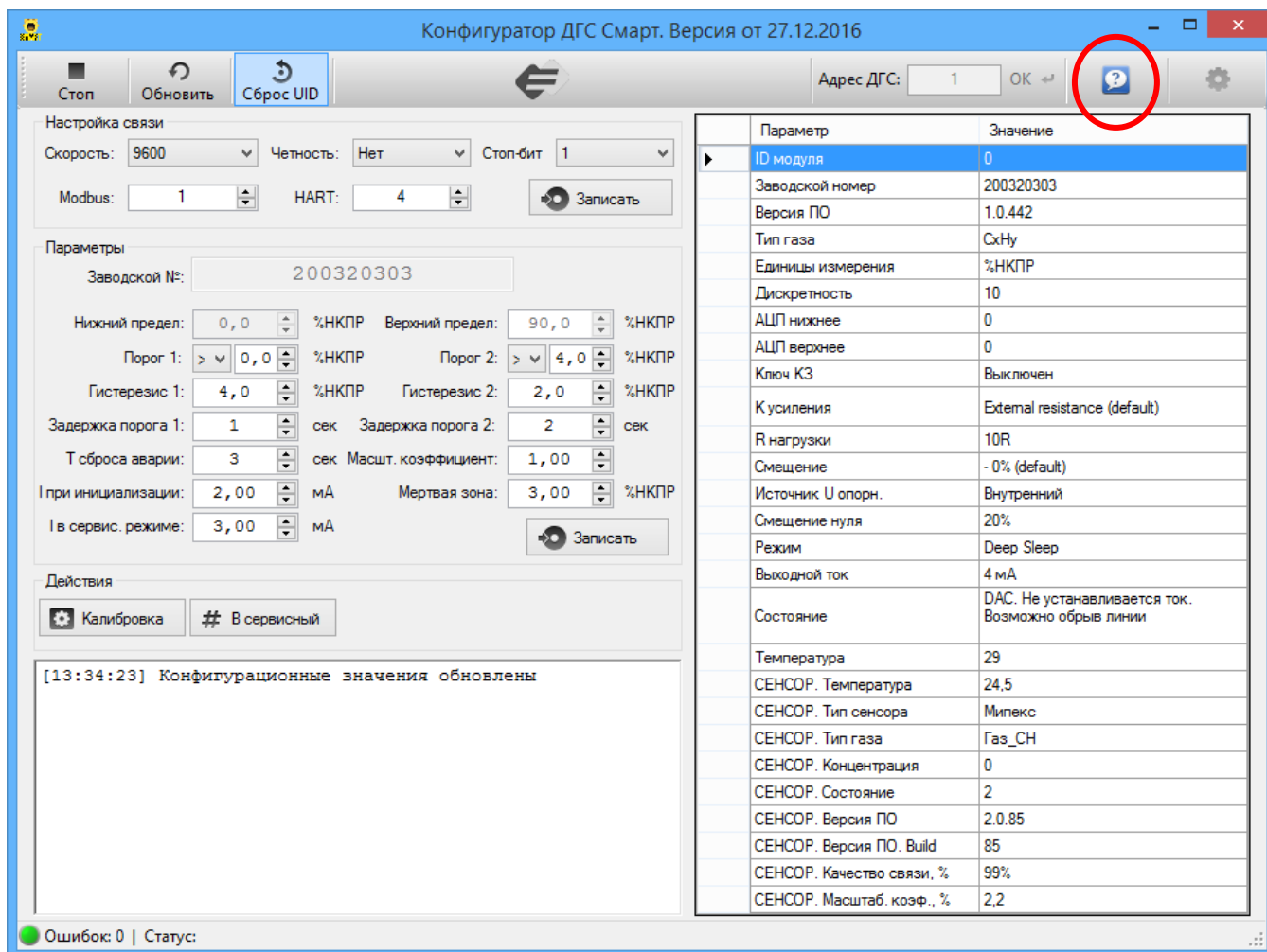
Рисунок Л.1- Главное окно ПО
