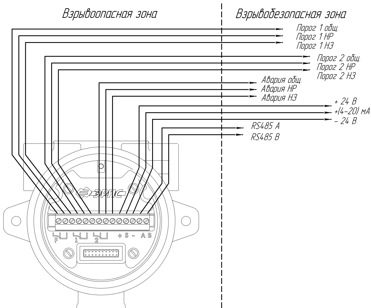
Рисунок Б.1 - Схема подключения газоанализатора ДГС ЭРИС-210 с реле
