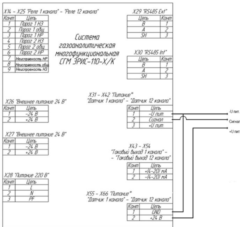
Рисунок Б.2 – Схема электрических подключений ЭРИС-110-А/К (для датчиков большой мощности)
