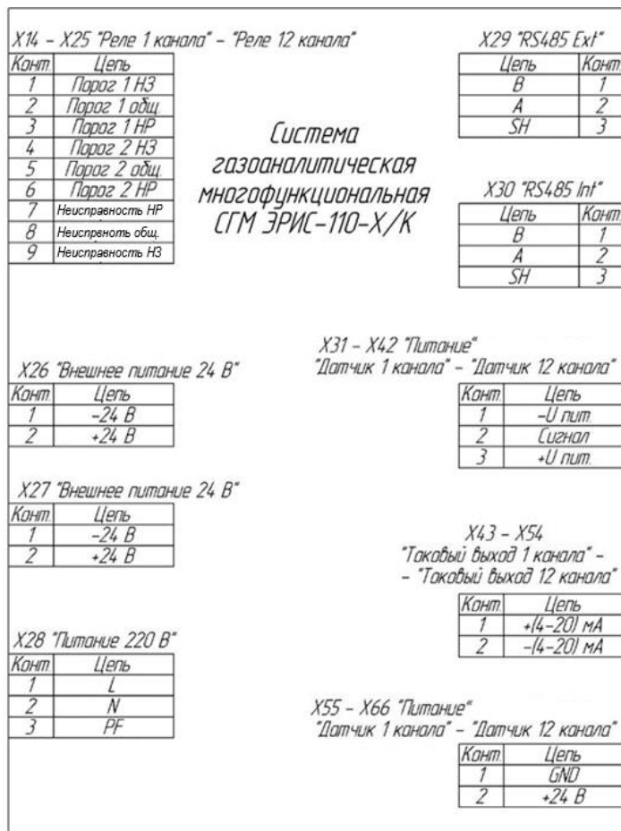
Рисунок Б.1 – Схема электрическая подключений ЭРИС -110-Х/К
