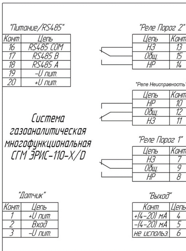
Рисунок Б.3 – Схема электрическая подключений ЭРИС -110-Х/D
