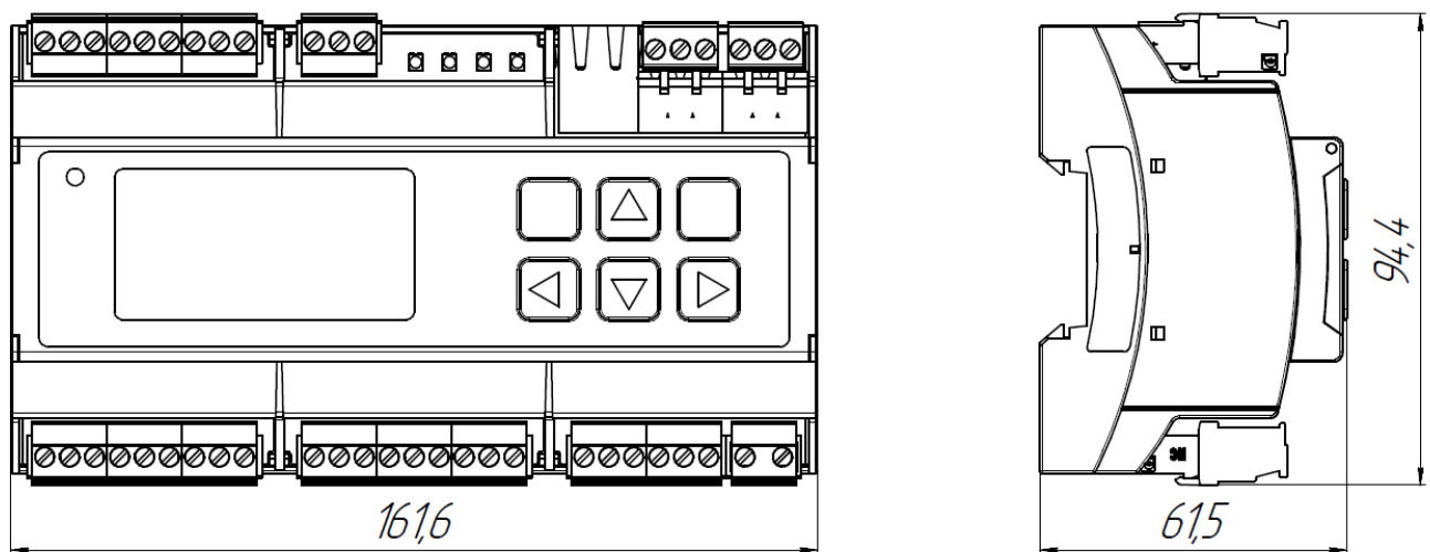
Рисунок В.2 – Габаритные и установочные размеры СГМ ЭРИС-110-Х/Д.
