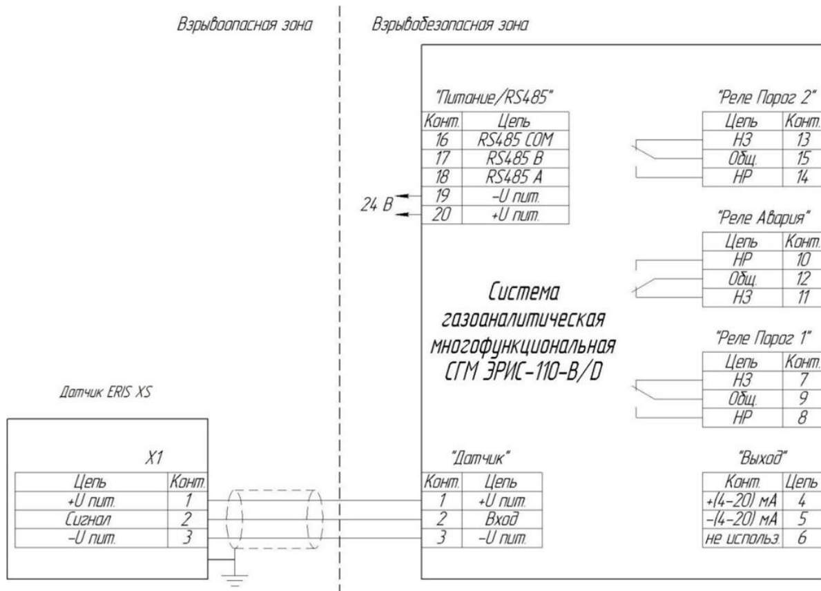
Рисунок Б.5 – Схема электрическая подключений ЭРИС -110-В/Д
