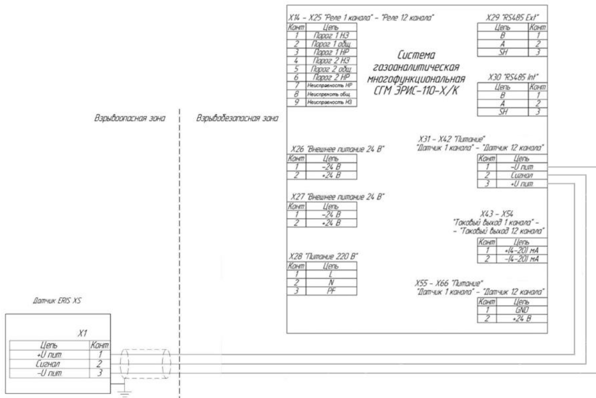
Рисунок Б.6 – Схема электрическая подключений ЭРИС -110-В/К
