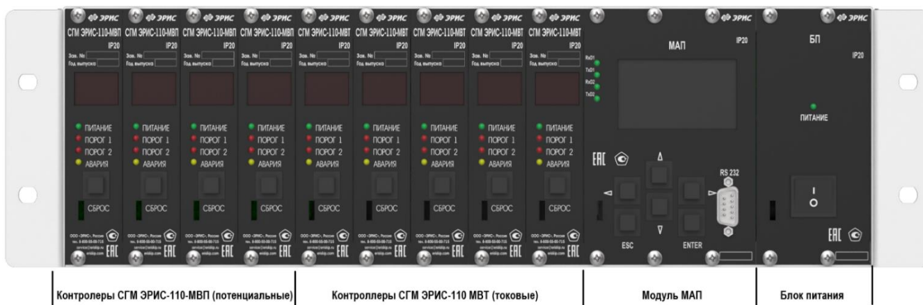
Рисунок 1 – Внешний вид системы СГМ ЭРИС-110- X/K
