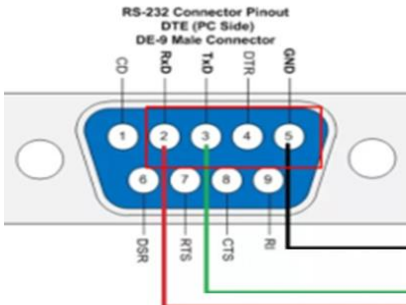
Рисунок 1 – Распиновка разъема на лицевой панели МАП.
