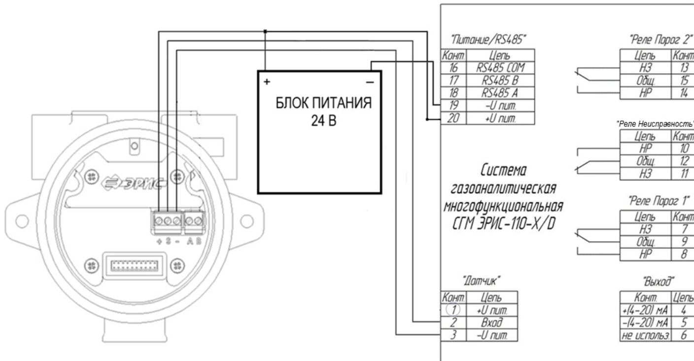
Рисунок Б.4 – Схема электрическая подключений ЭРИС -110-А/D с использованием дополнительного блока питания
