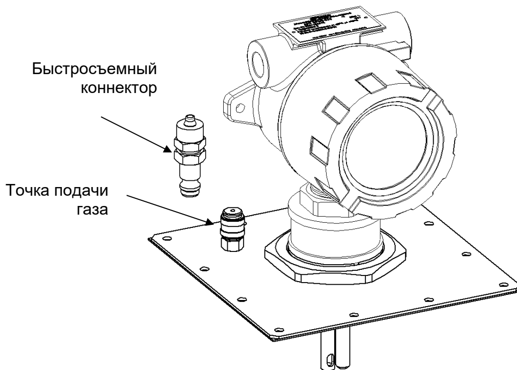
Рисунок 28 – Внешний вид газоанализатора и комплекта для монтажа в воздуховоде
