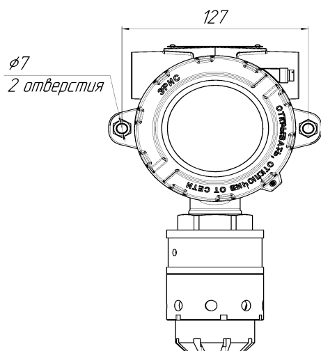
Рисунок 7 – Монтажные размеры
