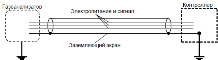
Рисунок 20 – Заземление экранированного кабеля
