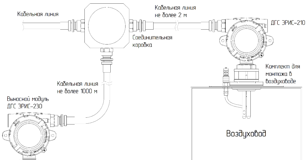
Рисунок 26 - Установка газоанализатора в воздуховоде с выносным модулем
