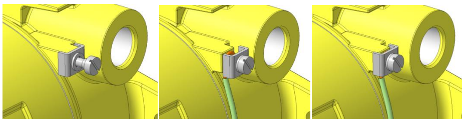
а) ослабить винт б) вставить провод в) затянуть винт Рисунок 21 – Заземление корпуса газоанализатора
