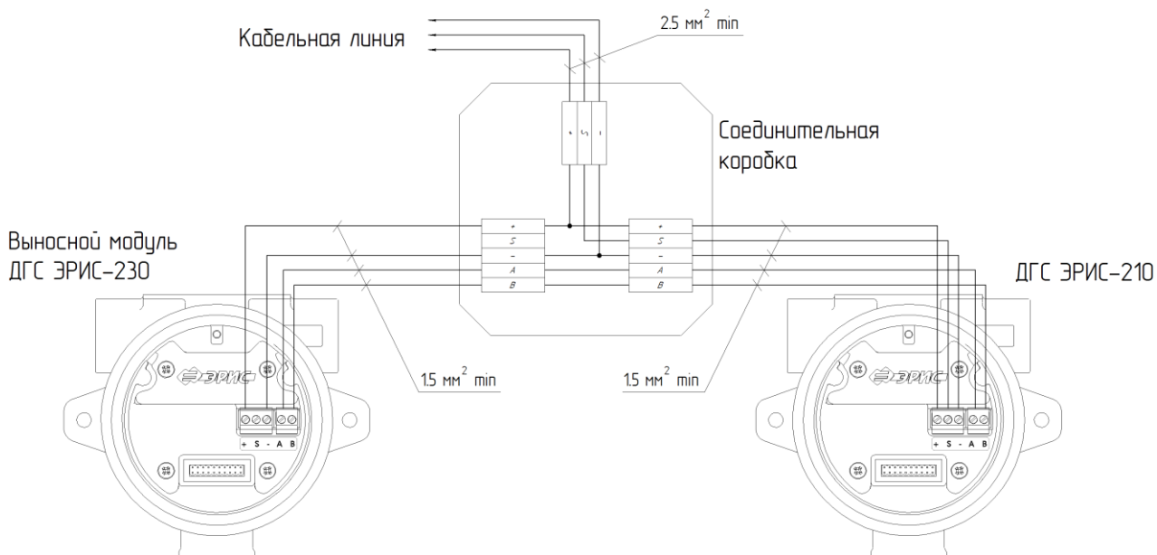
Рисунок 27 - Схема подключения выносного модуля и датчика ДГС ЭРИС-230
