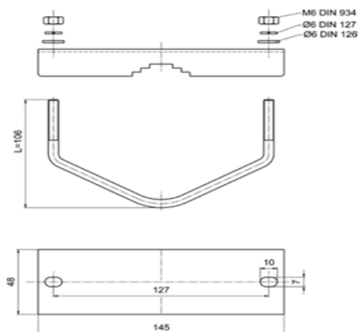
Рисунок 9 – Вид крепления для установки на трубу
