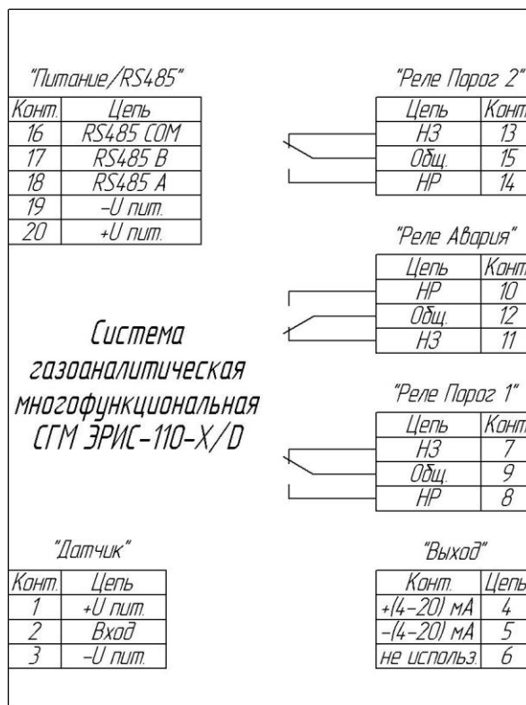
Рисунок Б.3 – Схема электрическая подключений ЭРИС -110-Х/Д
