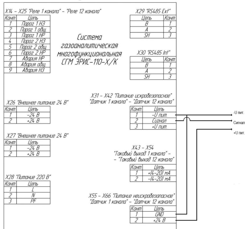
Рисунок Б.2 – Схема электрических подключений ЭРИС-110-Х/К (для датчиков большой мощности)
