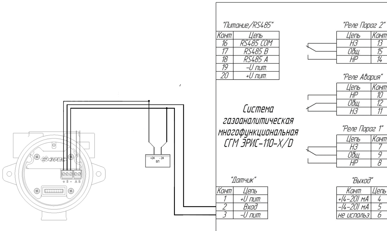
Рисунок Б.3 – Схема электрическая подключений ЭРИС -110-Х/Д
