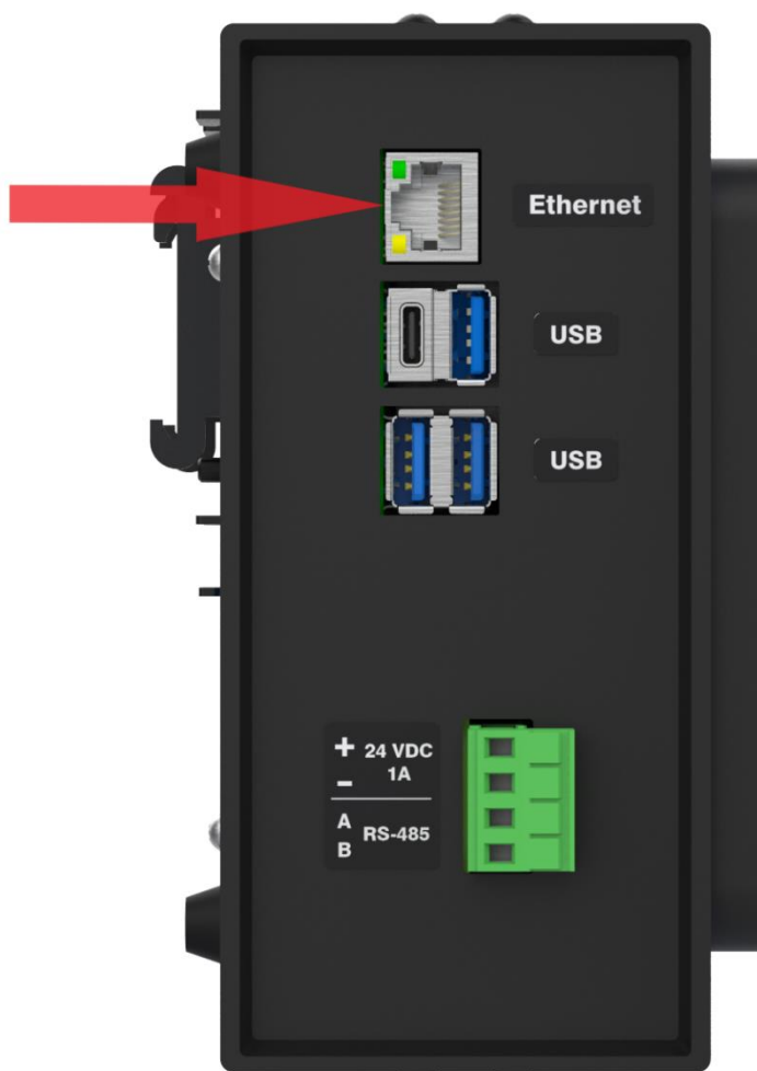
Рисунок В.2 – Подключение сетевого кабеля
