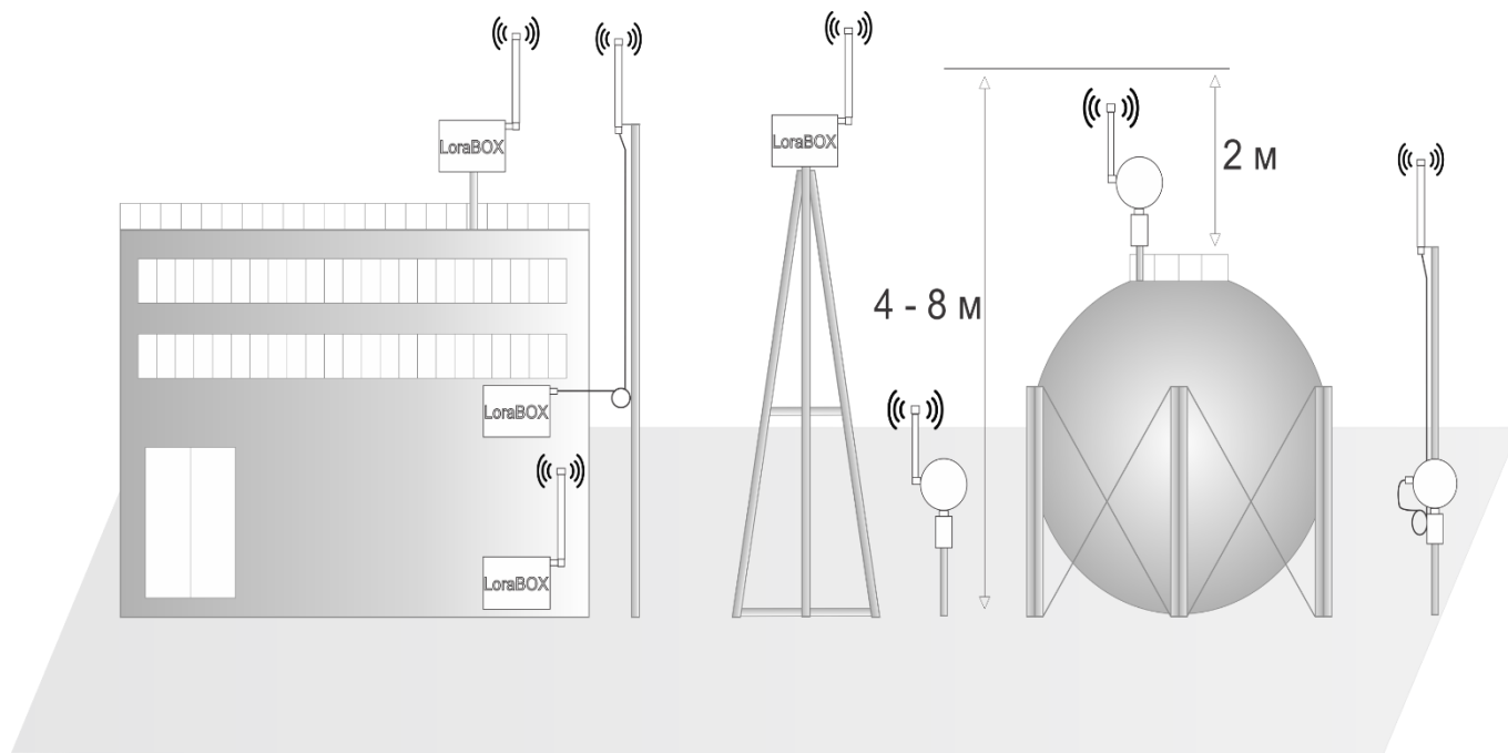
Рисунок 7 – Пример установки устройств
