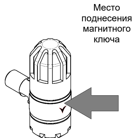
Рисунок 26 – Внешний вид газоанализатора со светозвуковым оповещателем С30
