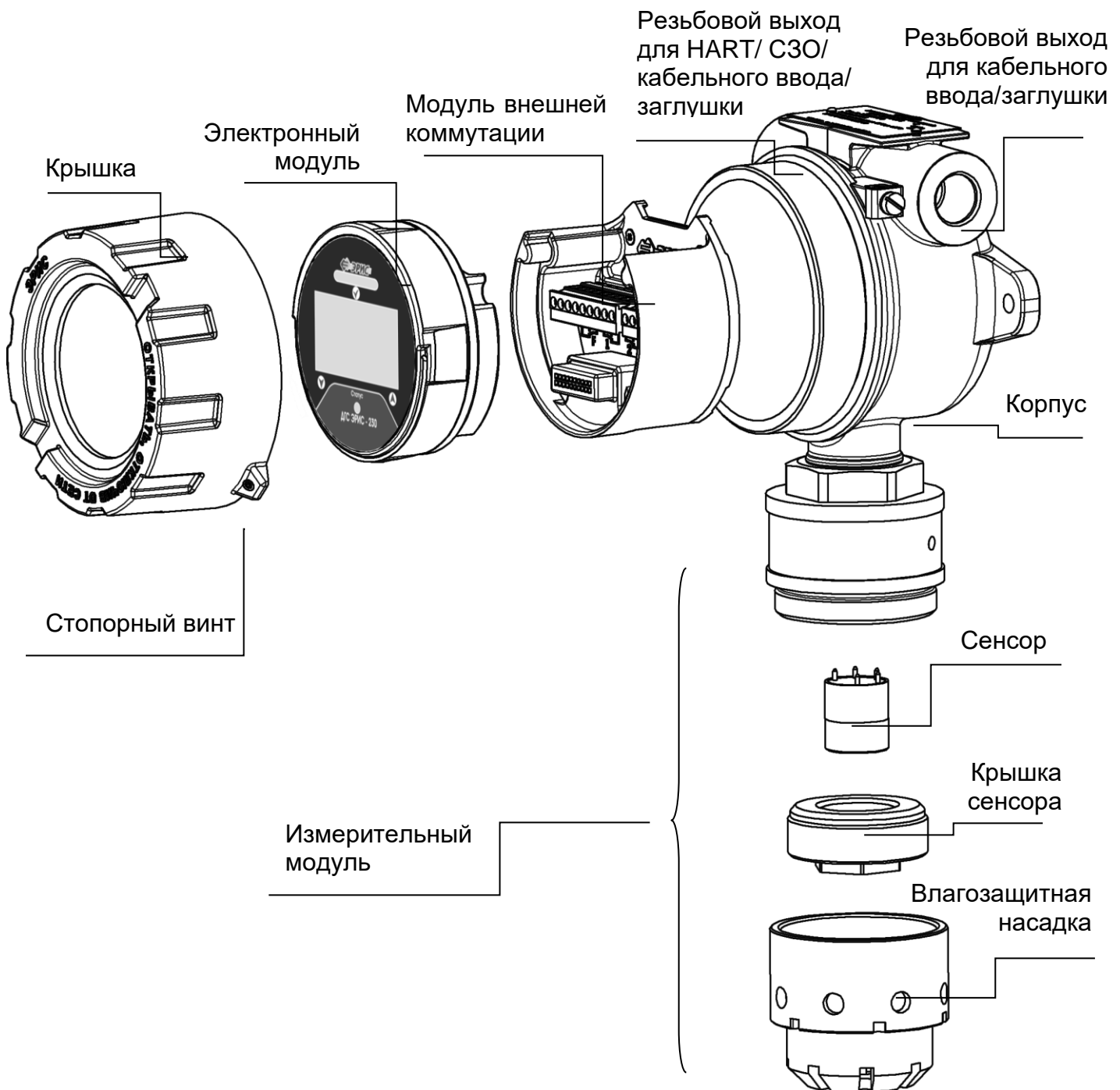
Рисунок 5 – Функциональный состав ДГС ЭРИС-230
