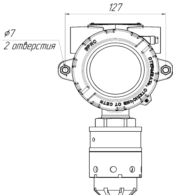
Рисунок 8 – Монтажные размеры
