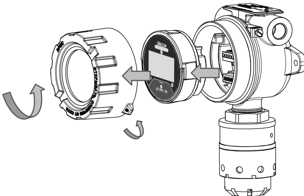
Рисунок 16 – Схема разбора ДГС ЭРИС-230
