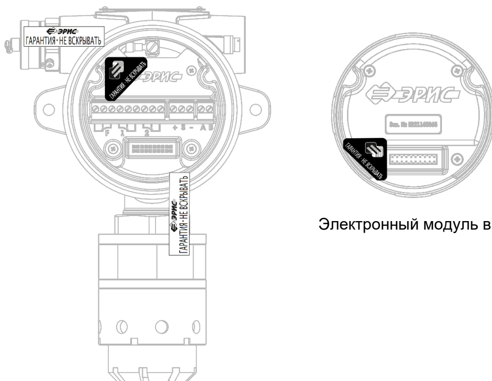
Рисунок 7 - Места нанесения пломб
