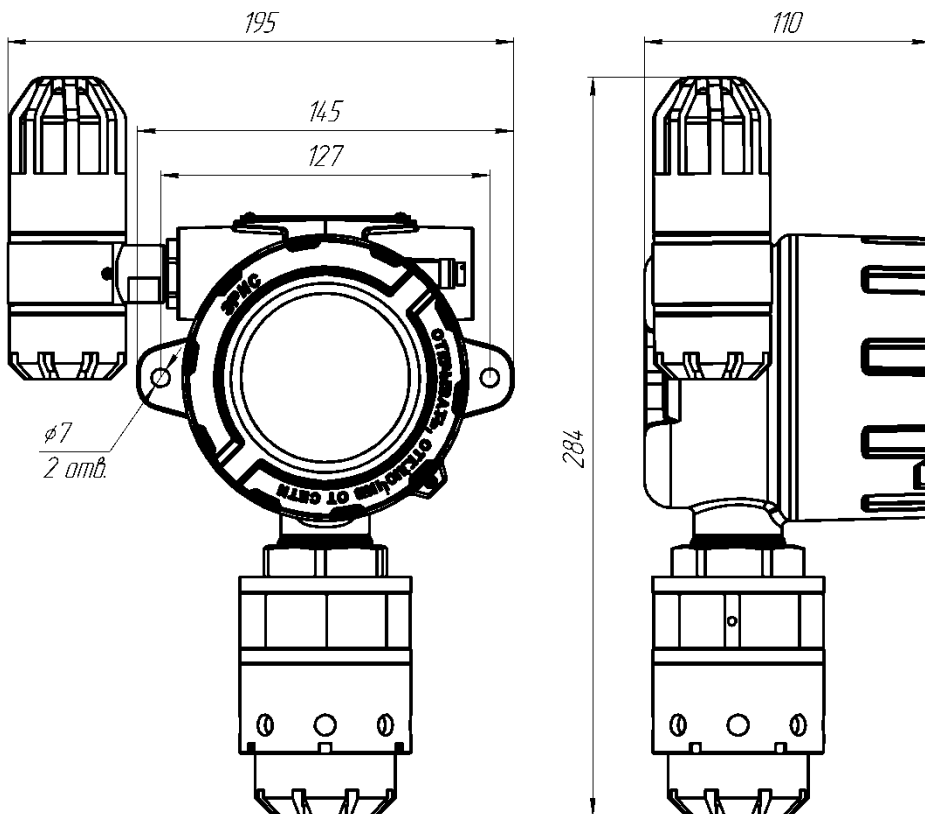
Рисунок 4 – Габаритные размеры ДГС ЭРИС-ФИД в комплектации со светозвуковым оповещателем СЗО
