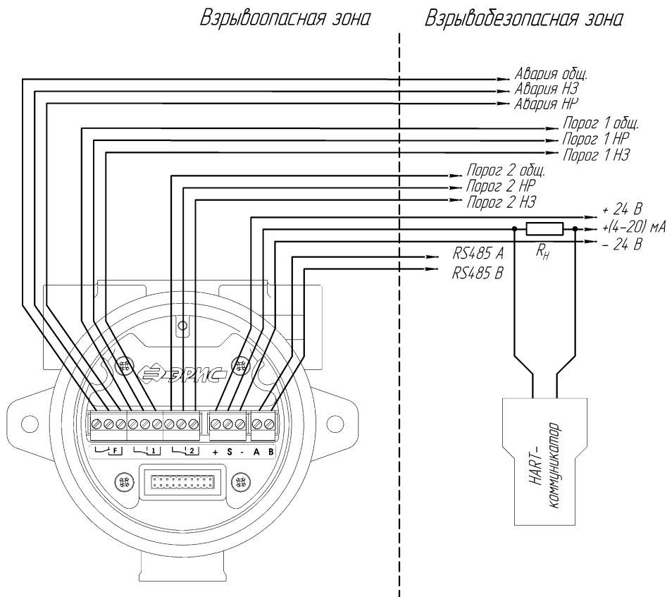
Рисунок 18 – 3-проводная схема подключения газоанализатора ДГС ЭРИС-ФИД с реле с подключением HART по токовой петле. НР - нормально разомкнутый контакт; НЗ - нормально замкнутый контакт.
