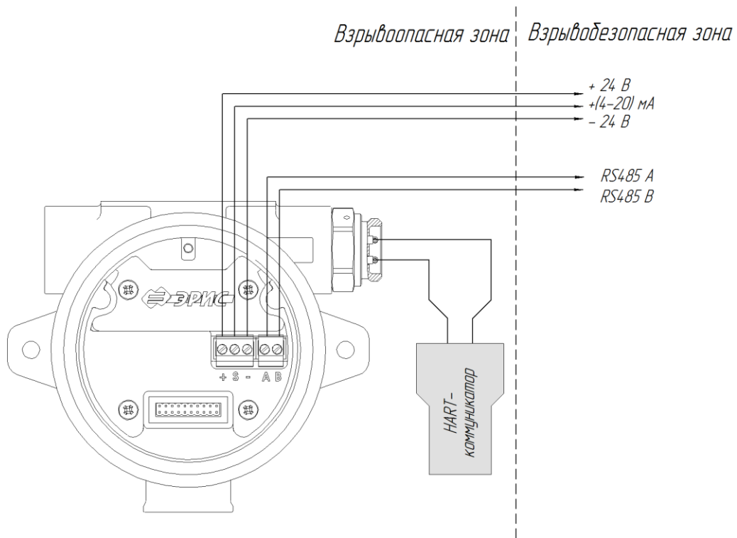
Рисунок 19 – 3-проводная схема подключения газоанализатора ДГС ЭРИС-ФИД без реле и с подключением локального HART
