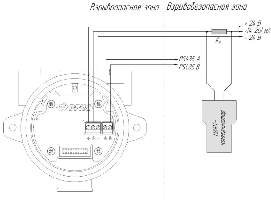
Рисунок 17 – 3-проводная схема подключения газоанализатора ДГС ЭРИС-ФИД без реле с подключением HART по токовой петле
