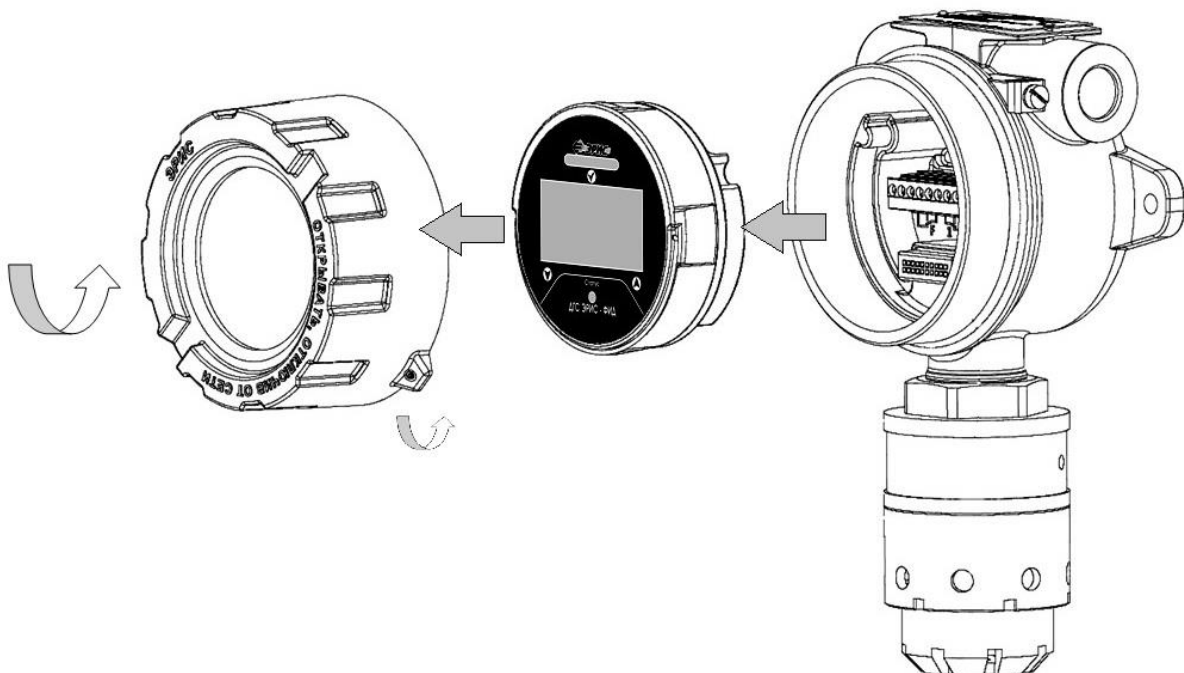
Рисунок 16 – Схема разбора ДГС ЭРИС-ФИД
