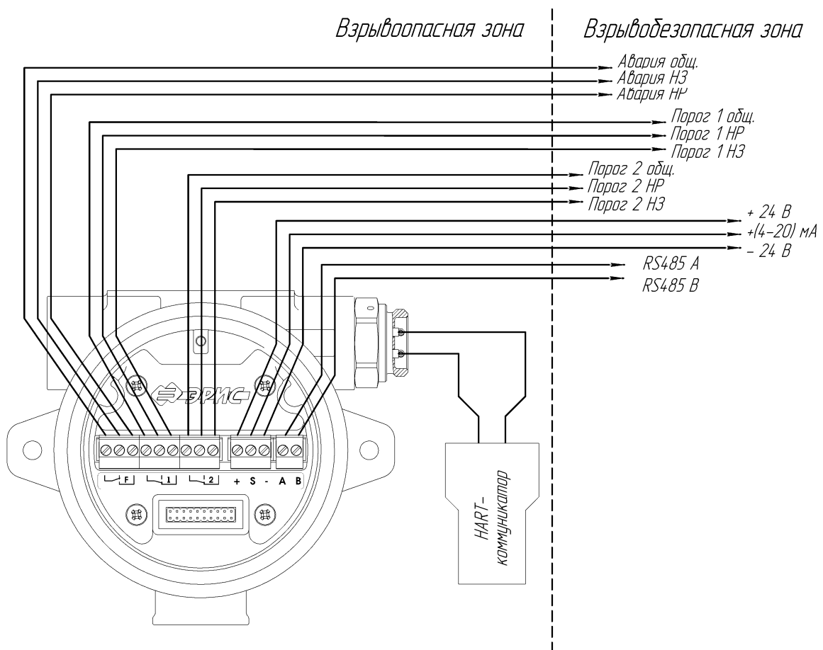
Рисунок 20 – 3-проводная схема подключения газоанализатора ДГС ЭРИС-ФИД с реле и подключением локального HART. НР - нормально разомкнутый контакт; НЗ - нормально замкнутый контакт.
