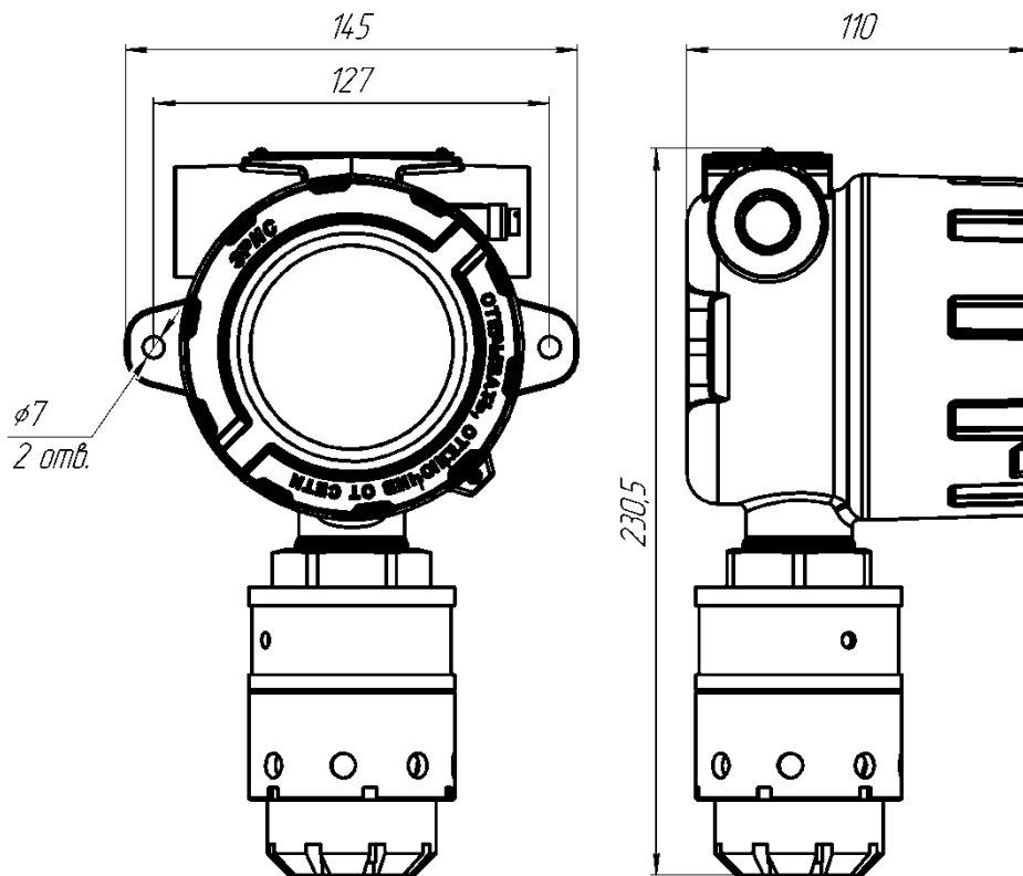
Рисунок 3 – Габаритные размеры ДГС ЭРИС-ФИД
