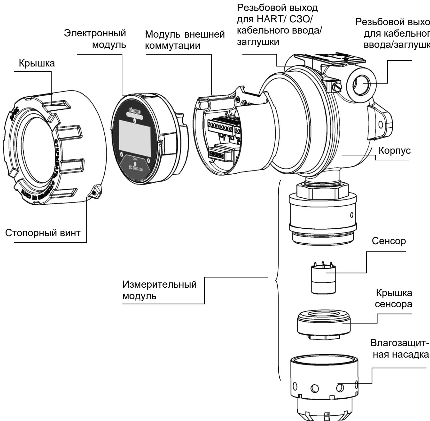
Рисунок 5 – Функциональный состав ДГС ЭРИС-ФИД М
