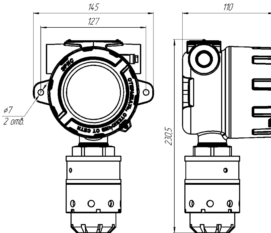
Рисунок 3 – Габаритные размеры ДГС ЭРИС-ФИД М
