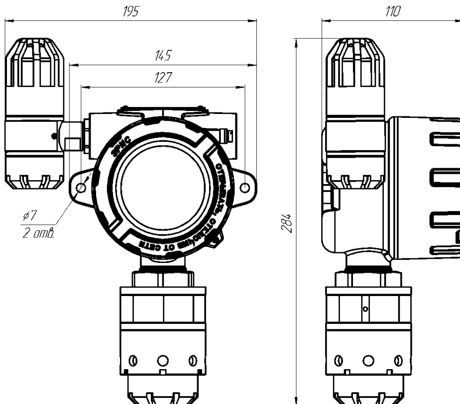
Рисунок 4 – Габаритные размеры ДГС ЭРИС-ФИД М в комплектации со светозвуковым оповещателем СЗО
