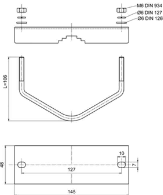
Рисунок 10 – Вид крепления для установки на трубу
