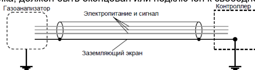
Рисунок 21 – Заземление экранированного кабеля
