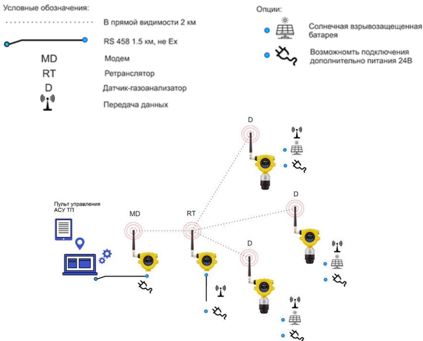
Рисунок 5 - Схема работы беспроводных устройств
