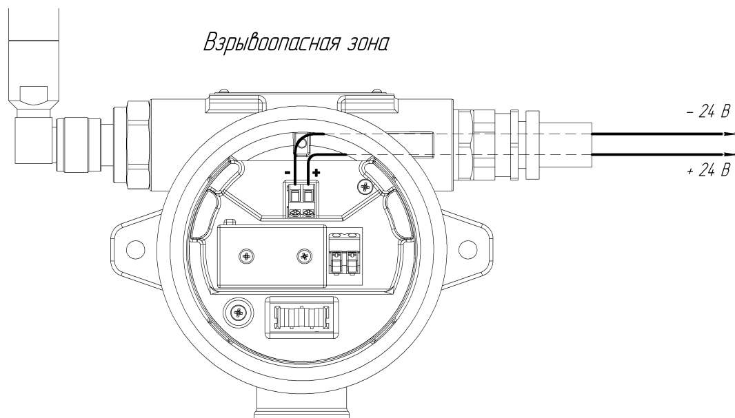
Рисунок 17 – Схема подключения газоанализатора
