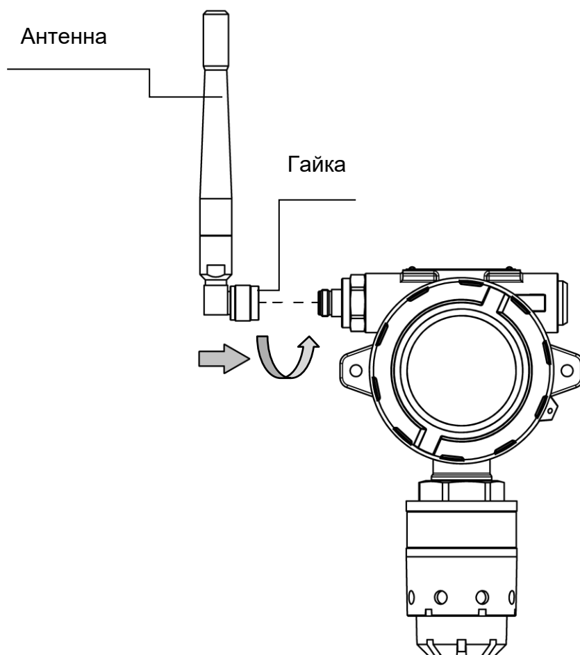
Рисунок 6 – Установка антенны
