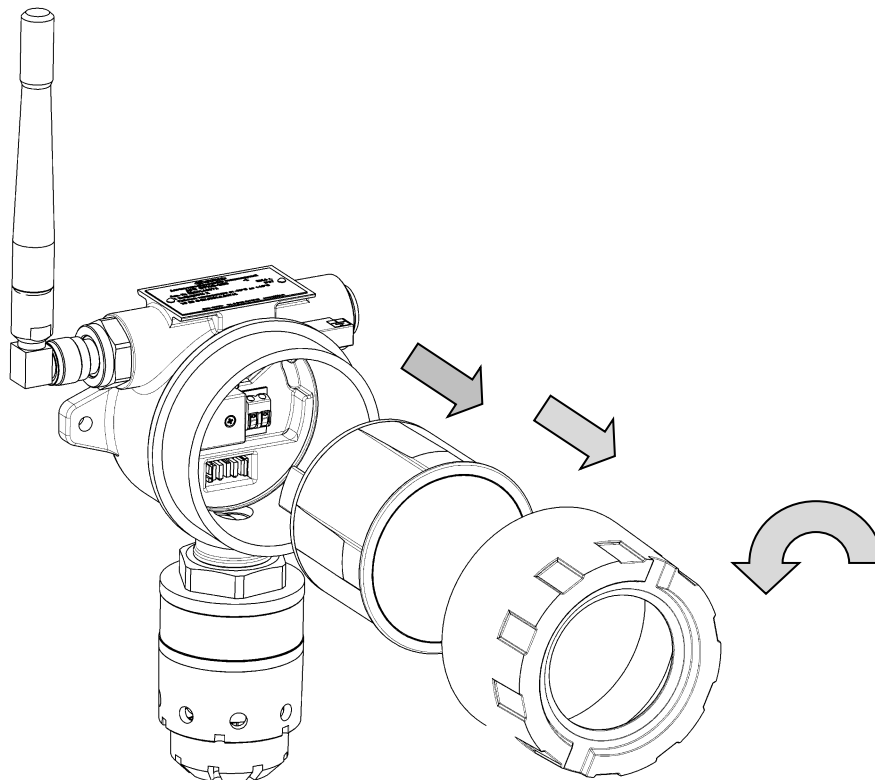
Рисунок 16 – Схема разбора ДГС ЭРИС-210
