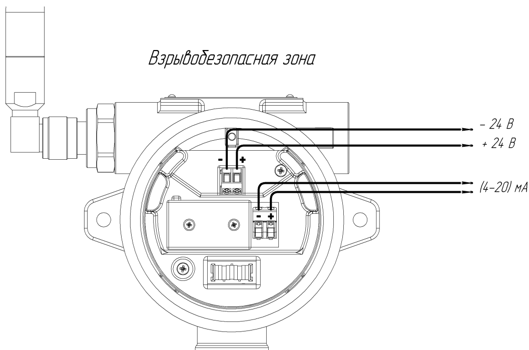
Рисунок 18 – Схема подключения газоанализатора в лабораторных условиях
