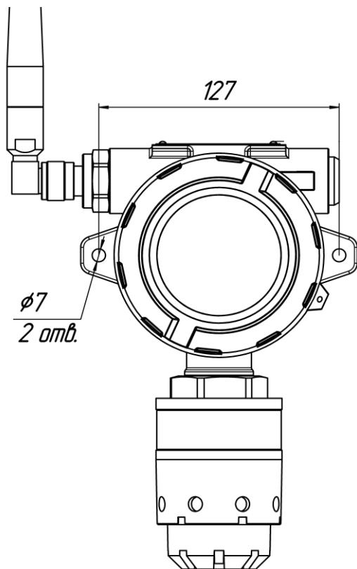
Рисунок 9 – Монтажные размеры
