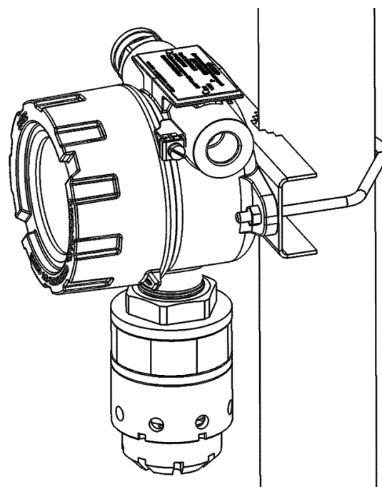
Рисунок 12 – Вид газоанализатора, установленного на трубу (антенна условно не показана)
